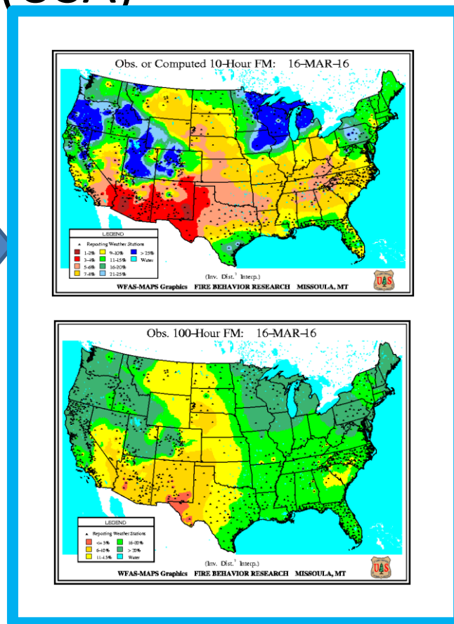
Índices de sequia de combustibles
